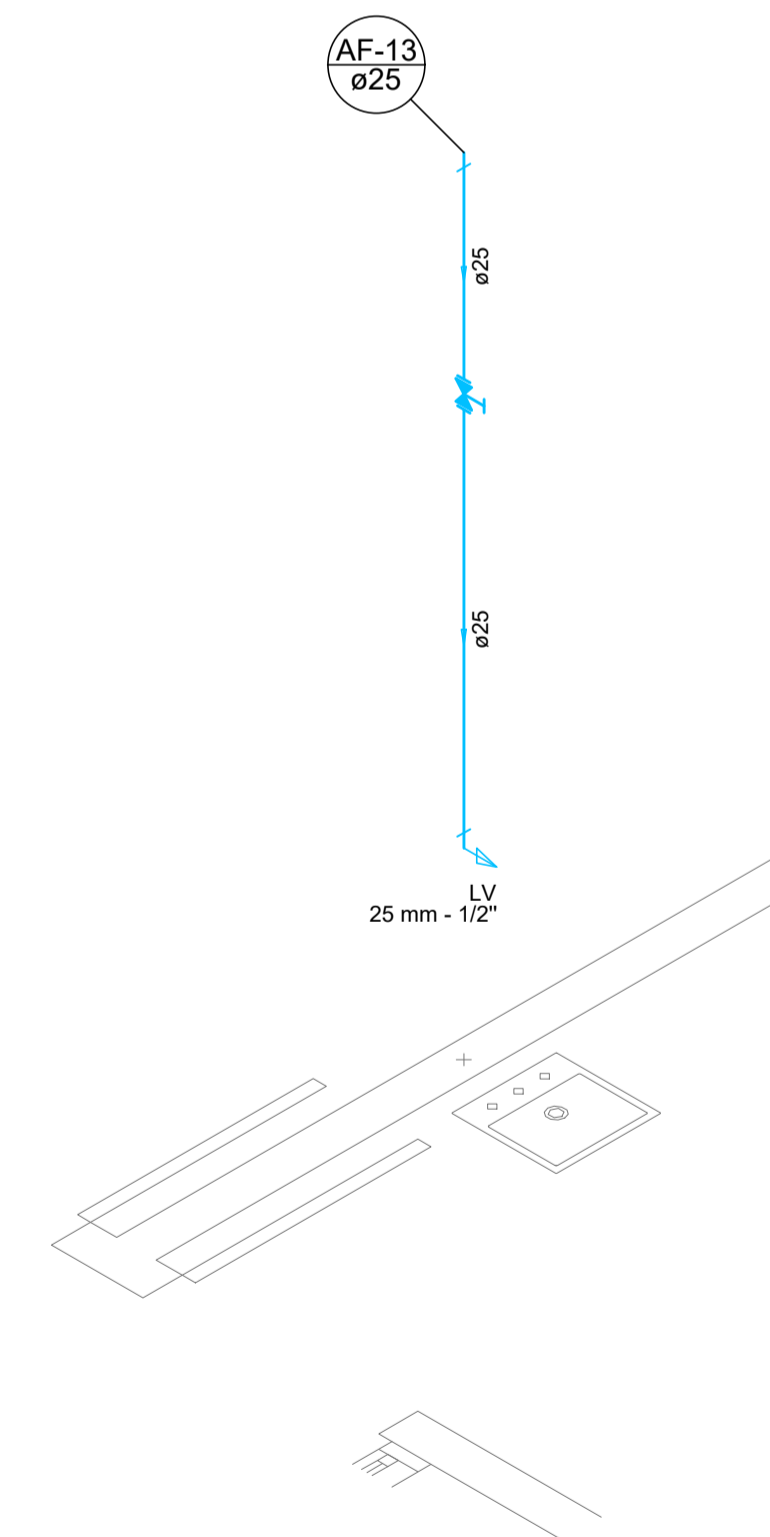
Detalhe H-12 Escala 1:25
