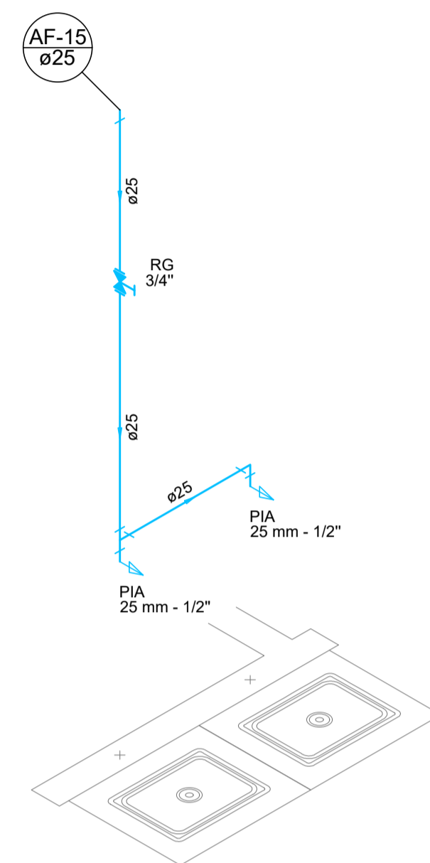
Detalhe H-14 Escala 1:25
