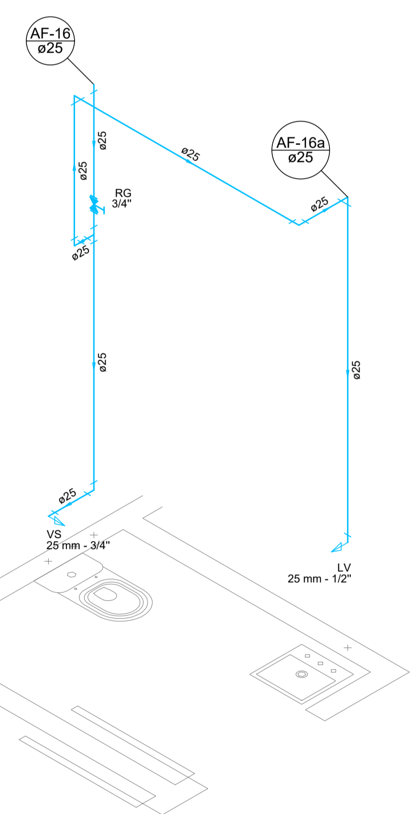
Detalhe H-14 Escala 1:25
