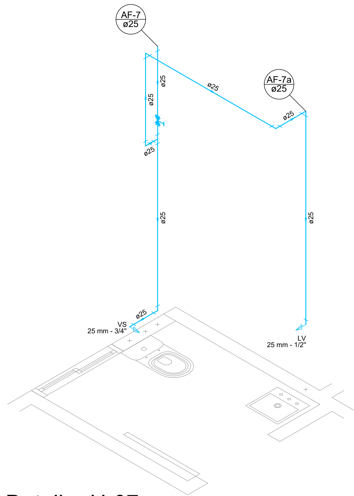
Detalhe H-07 Escala 1:25
