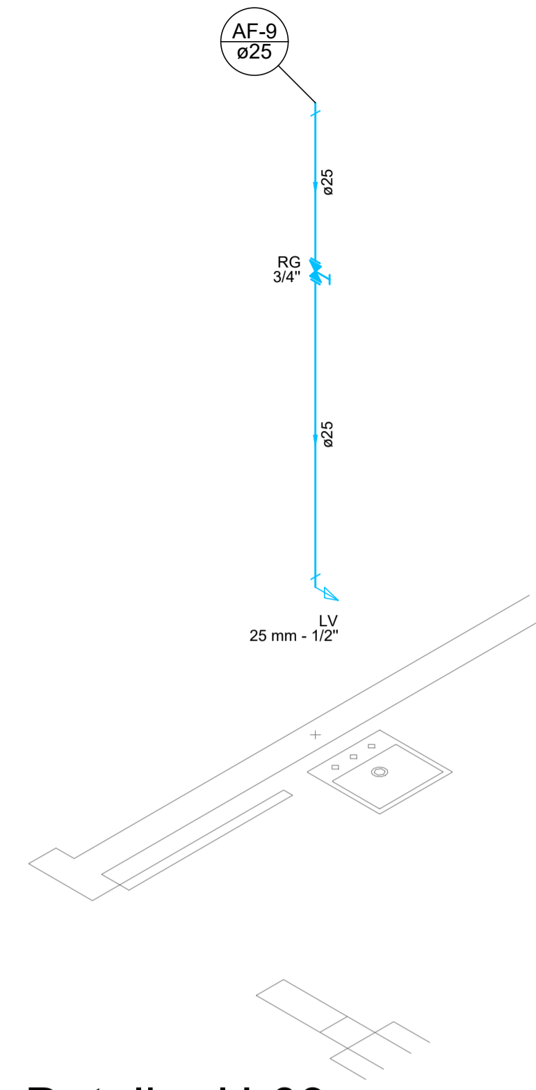
Detalhe H-09 Escala 1:25
