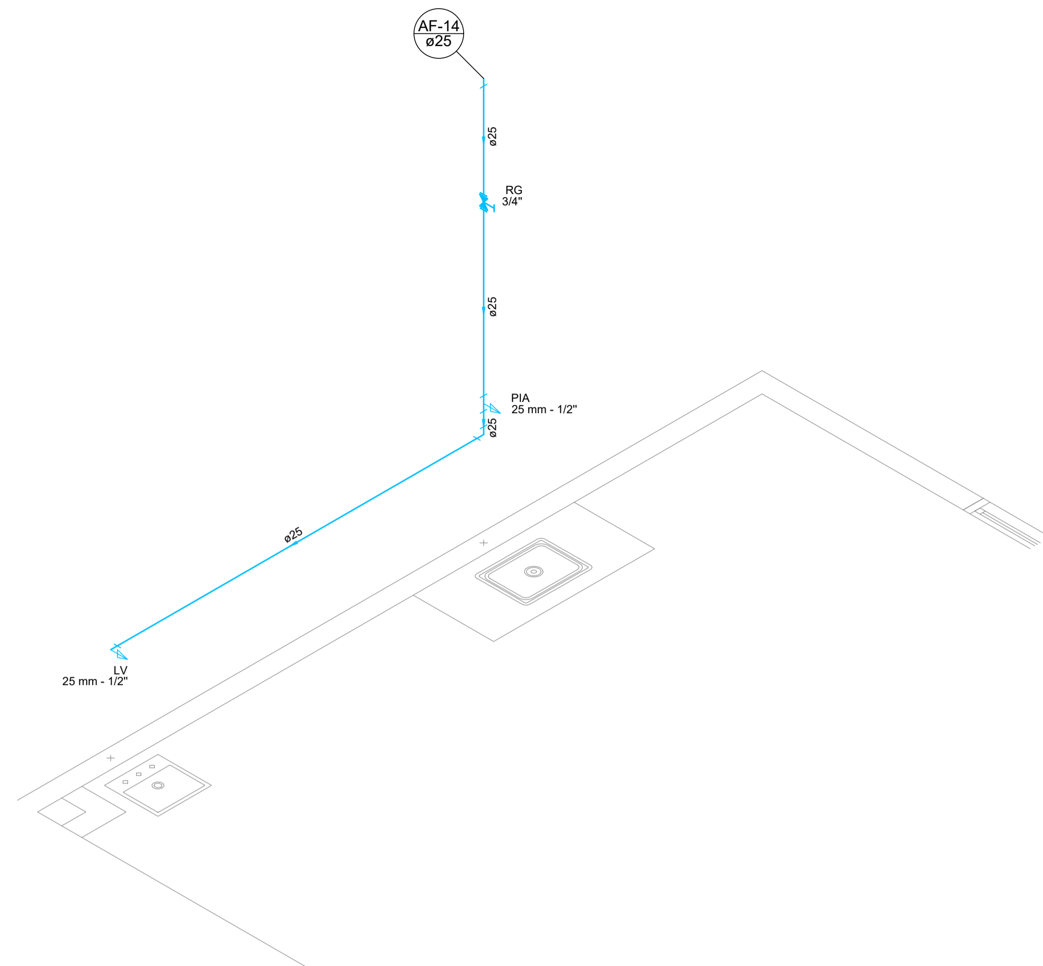
Detalhe H-13 Escala 1:25
