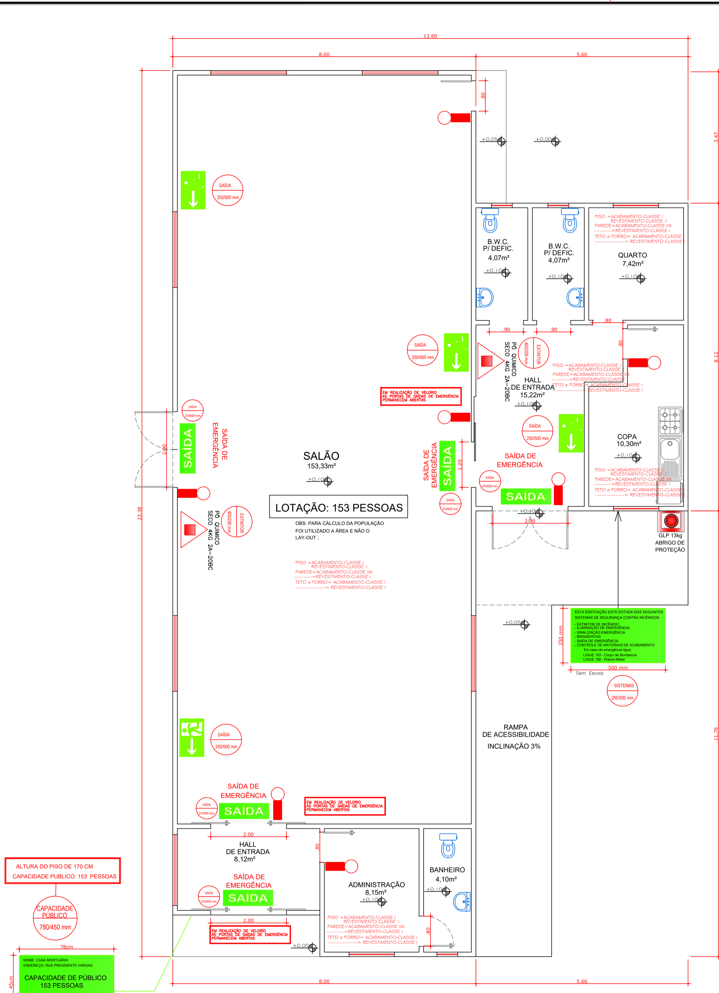
PLANTA BAIXA ESCALA - 1:50 ÁREA 248,12m²
