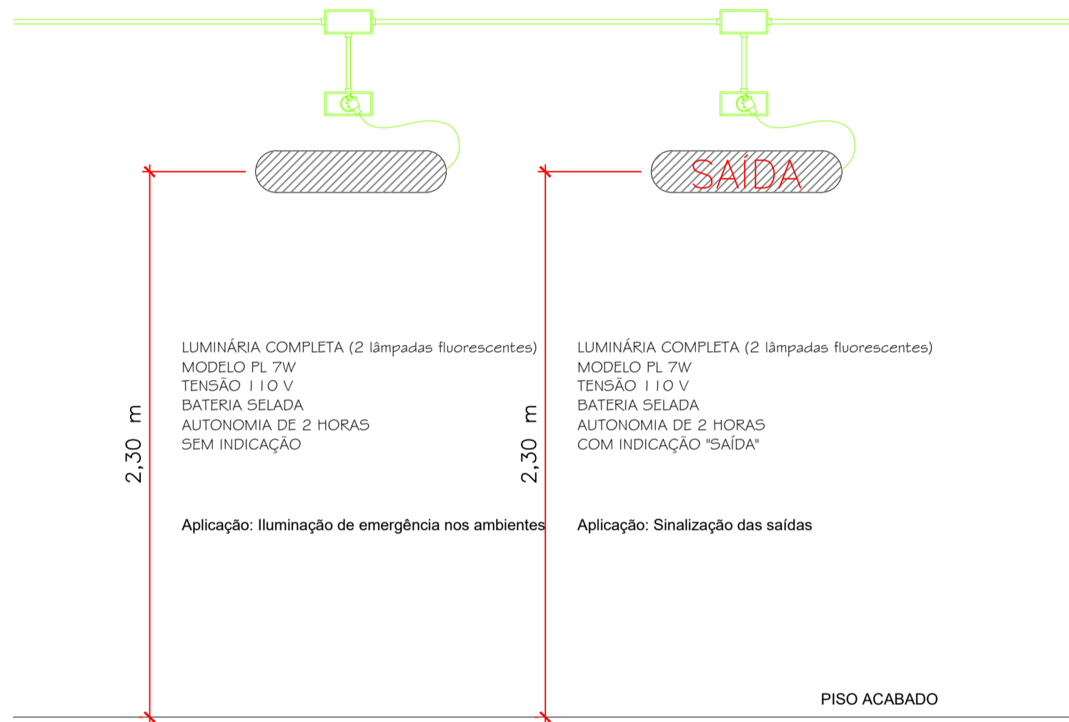
DETALHE Luminárias de Emergência
