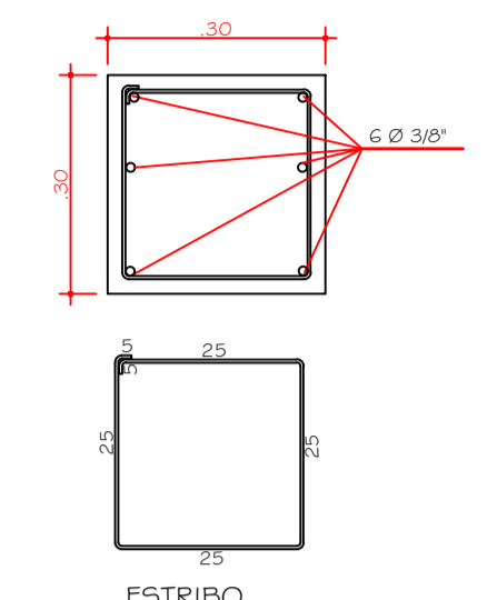
PLANTA DOS PILARES / I 9-20-2 I ESCALA 1: 10 TOTAL DE PILARES=3 PILARES(30x30x4,00)= 3X
