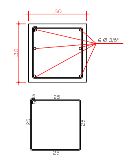
VIGA DETALHE -VDT 30X30 ESCALA 1: 10 TOTAL DE VIGAS=3 VIGAS DO DETALHE(30x30x4,00)= 3X
