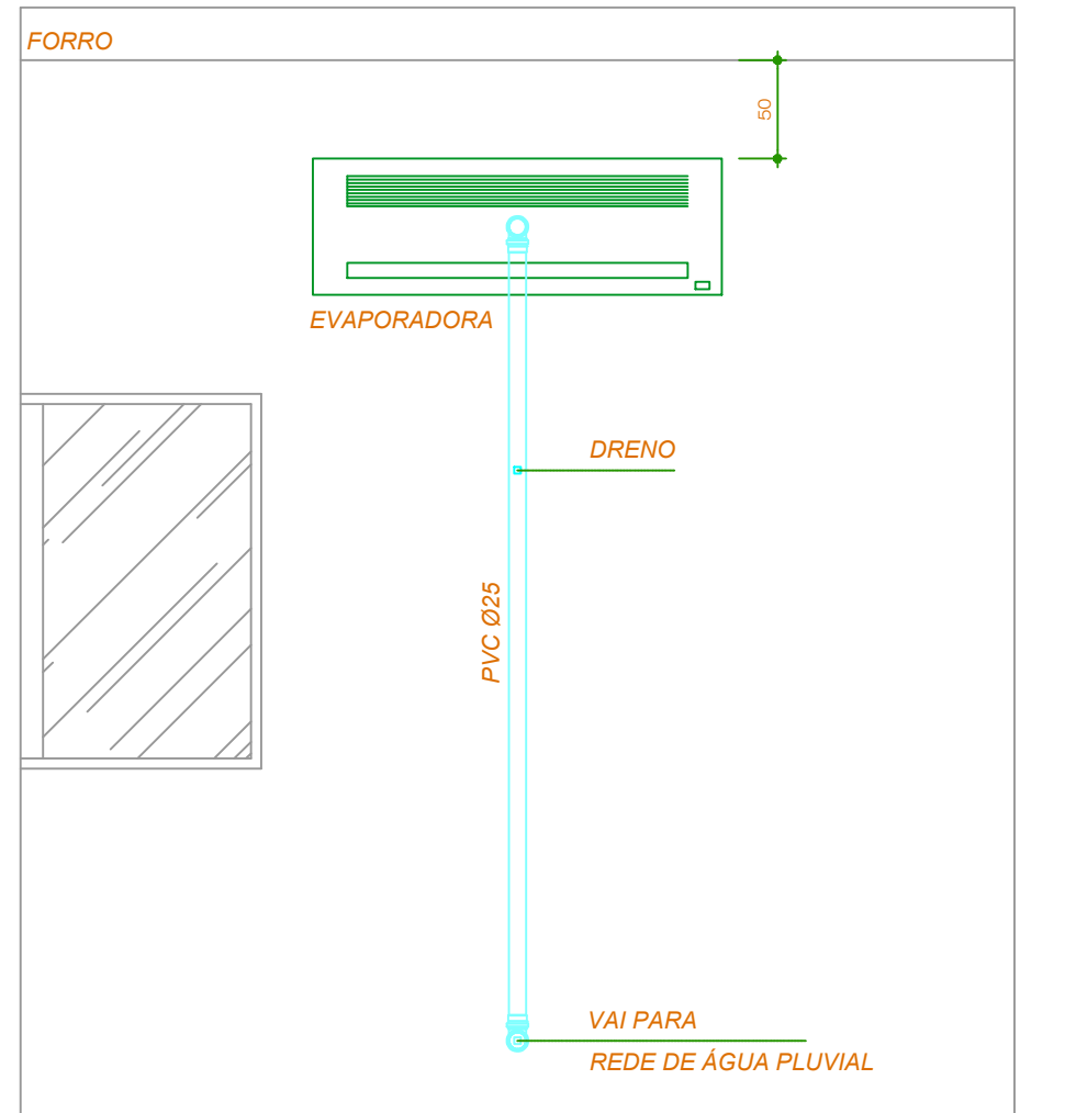
02 DETALHE - DRENO EVAPORADORA SEM ESCALA
